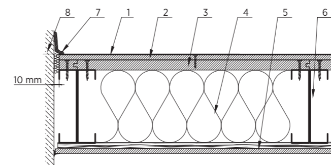
Rys 7. Detal wykończenia podkładu podłogowego wzdłuż ściany (Opis: 1. Warstwy wykończeniowe podłogi, 2. Płyty Cementex, 3. Płyty Duripanel, 4. Materiał izolacyjny, 5. Zabudowa sufitowa, 6. Nośna konstrukcja stalowa C254, 7. Listwa podłogowa, 8. Ściana)
