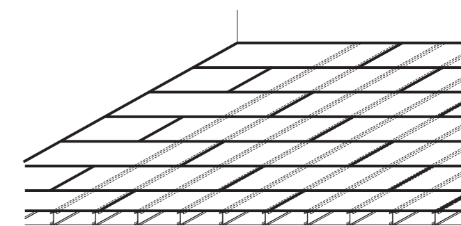
Rys 3. Schemat układu płyt Duripanel na konstrukcji
