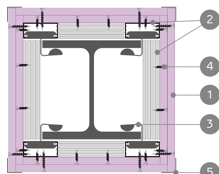
Klips mocujący KM do profili Nida CD60
