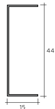
Profil sufitowy NIDA MFCC44 Grubość blachy 0,7 mm ocynk Z100
