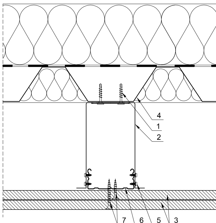
PRZEKRÓJ PIONOWY
